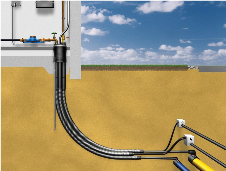
Bild 8: Mehrspartenhauseinführung für Gebäude ohne Keller*
