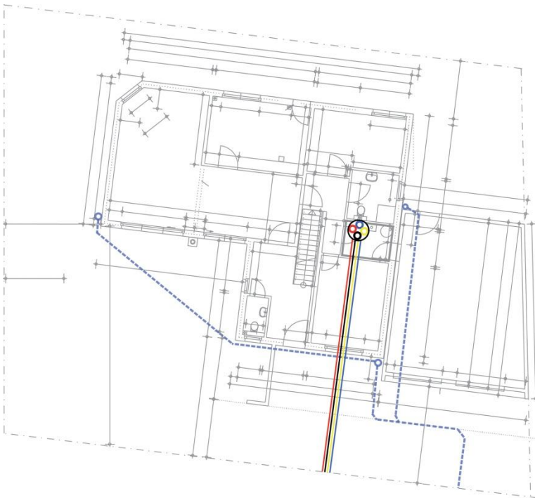
Bild 5: Ausführungsplan mit Mehrspartenhauseinführung*
