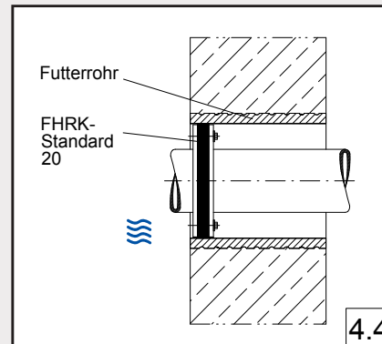
Wandeführung Betonwand mit Futterrohr
