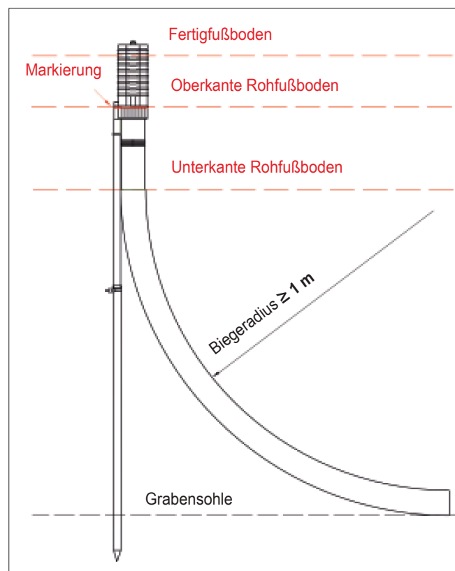
Mehrsparten-Hauseinführung
