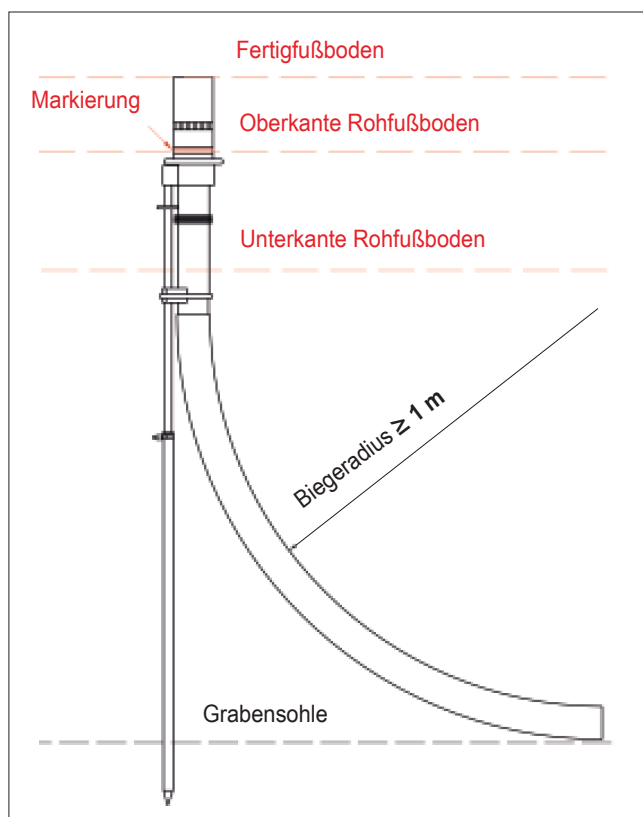
Einsparten-Hauseinführung
