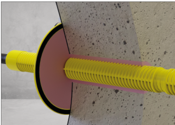
Wandeführung mit Vergussmörtel/ Expansionsharz und Dichtungsflansch
